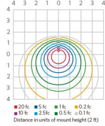
TD 9LED ISOFOOTCANDLE PLOT
